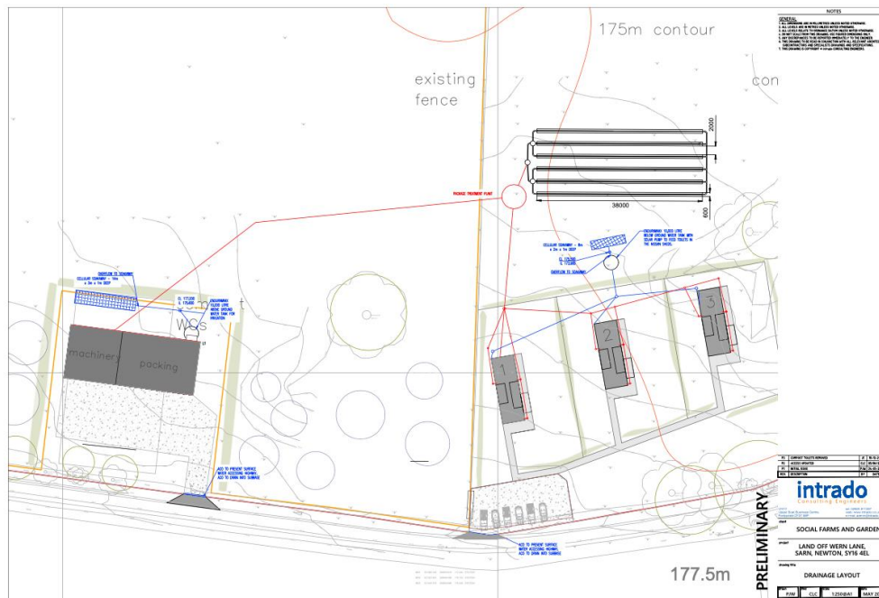
Cynllun SuDS / draenio cychwynnol
